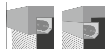
Pose en applique intérieure
